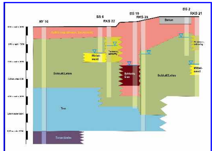
Geotechnischer Profilschnitt
