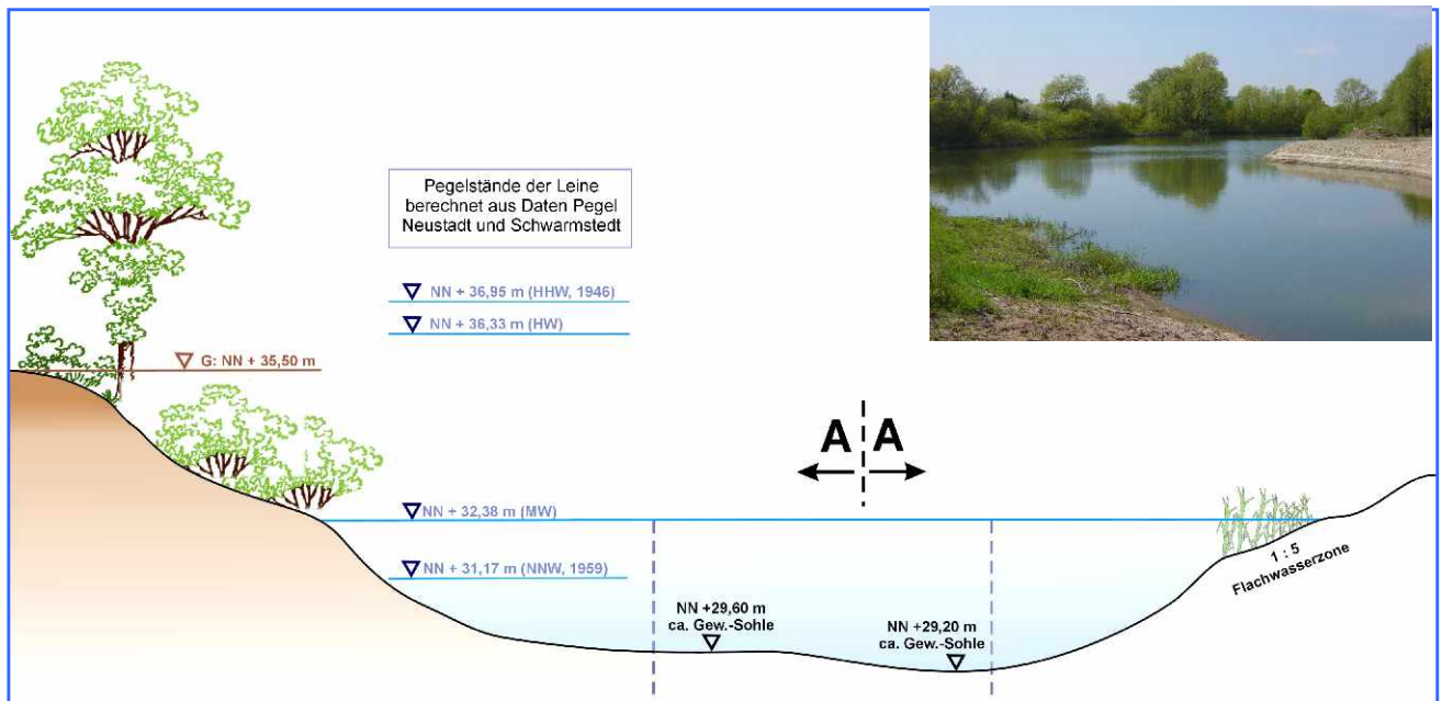
Längsschnitt (mit 10-facher Überhöhung)
