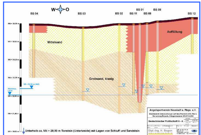
Geotechnischer Profilschnitt
