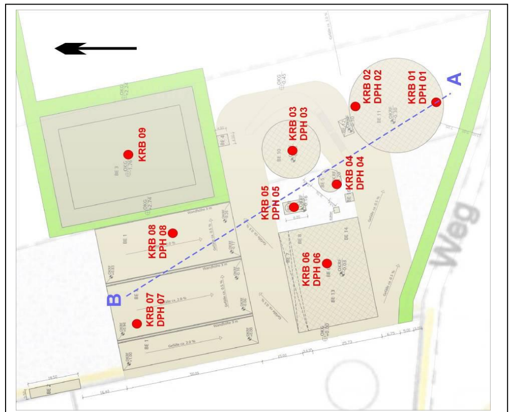
Lageplan der Kleinrammbohrungen und schweren Rammsondierungen und Achse A – B des geotechnischen Profilschnitts
