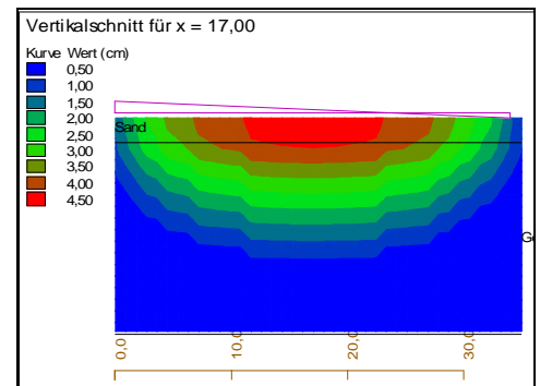
Schnitt durch den Baugrund unter einem der Großbehälter mit den zu erwartenden Setzungen
